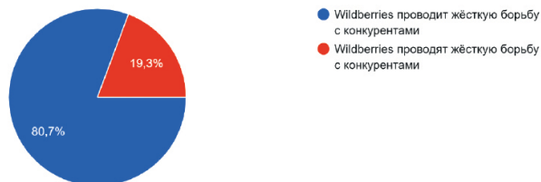
Рис. 4. Согласование между субъектом и предикатом в настоящем времени
