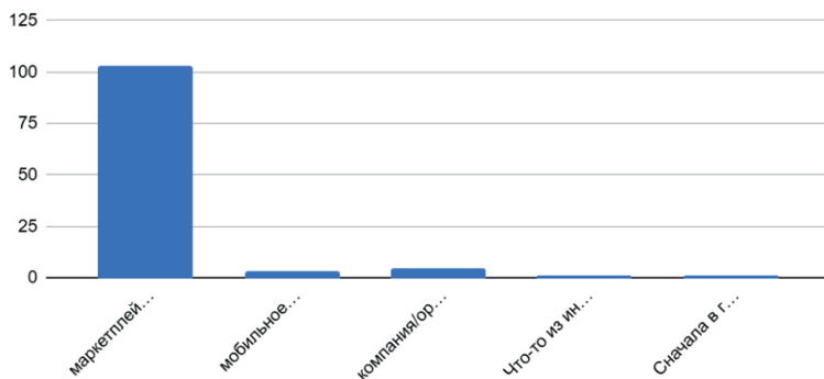
Рис. 3. Соотнесение онима с денотатом
